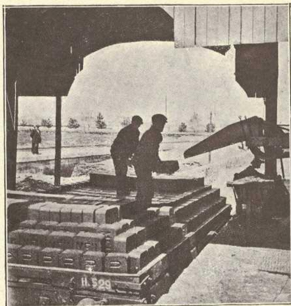
Fábrica de briqueta: salida del producto
