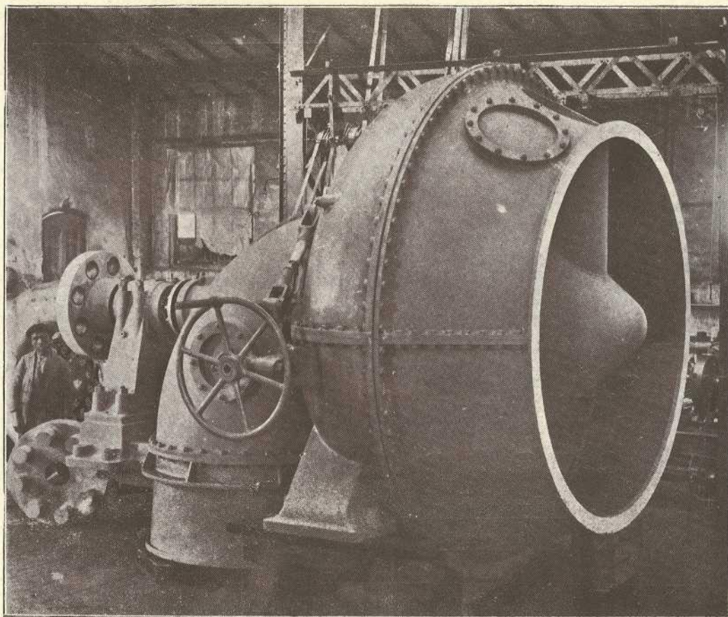
Turbina de eje horizontal con cámara, entrada axial, para 730 C. V.
