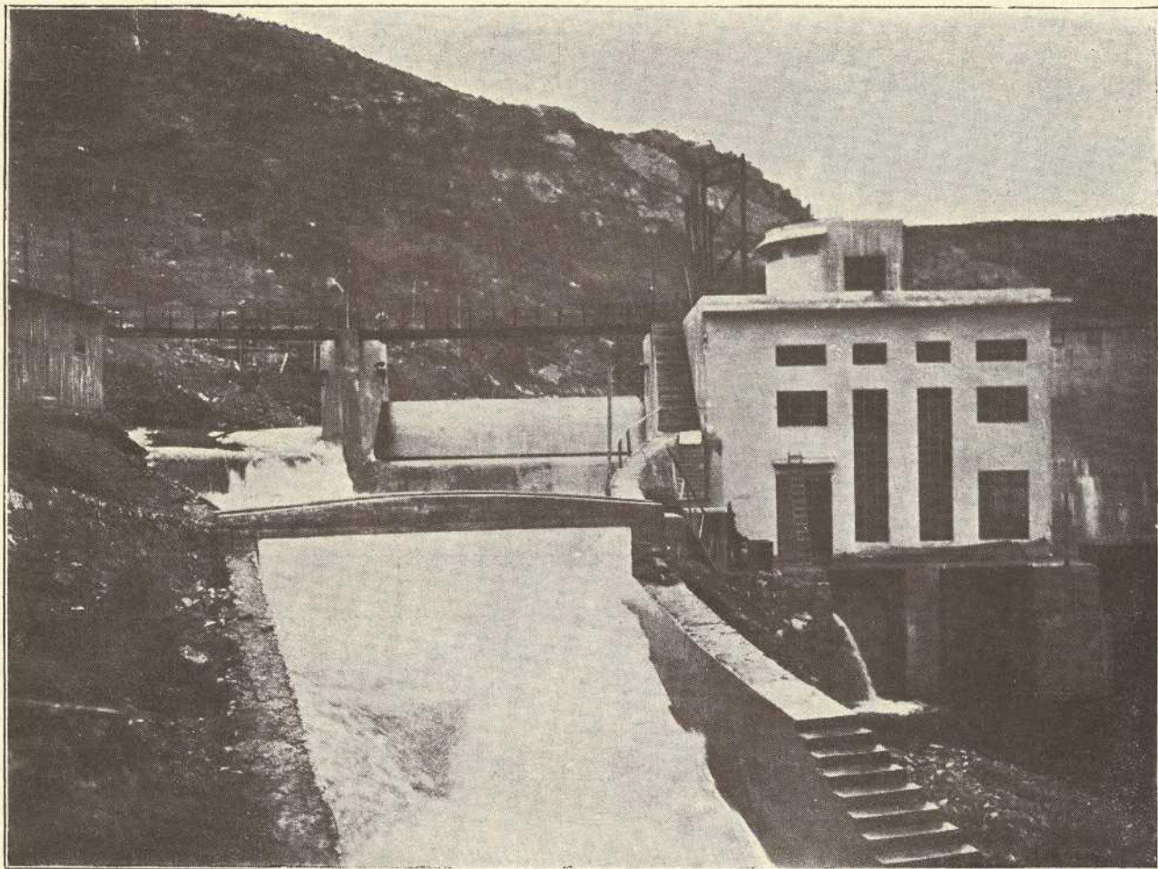
"El Irati" S. A., Pamplona. — Dos alzas automáticas de sector metálico de 13 m. y 11 m. ancho y 3'50 m. altura instaladas en su salto de Usoz por Maquinaria y Metalurgia Aragonesa
